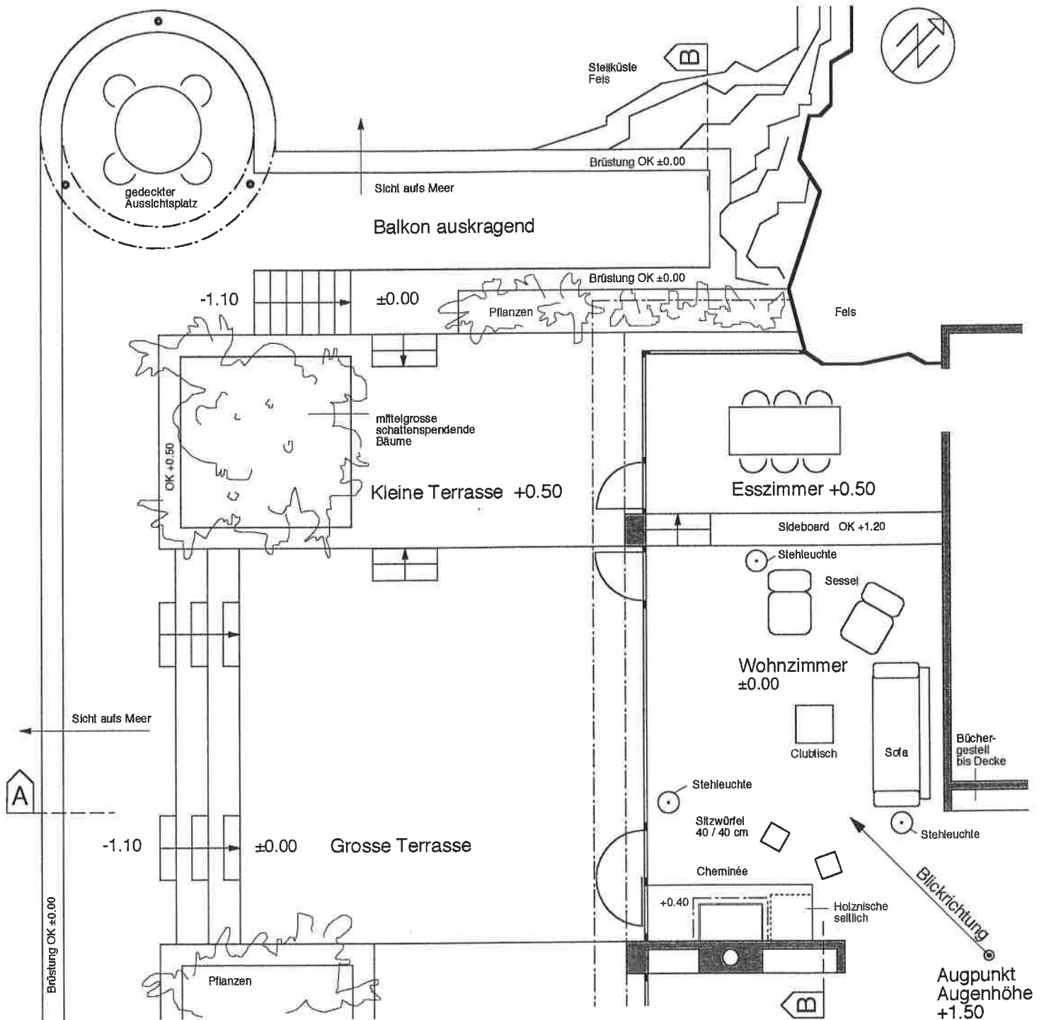
Grundriss 1:100
