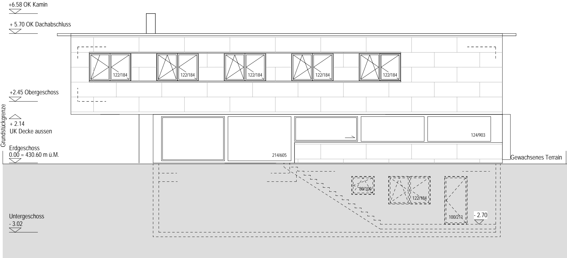
OSTANSICHT
