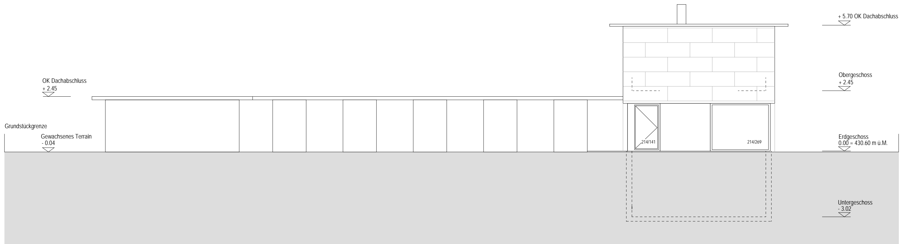
SÜDANSICHT
