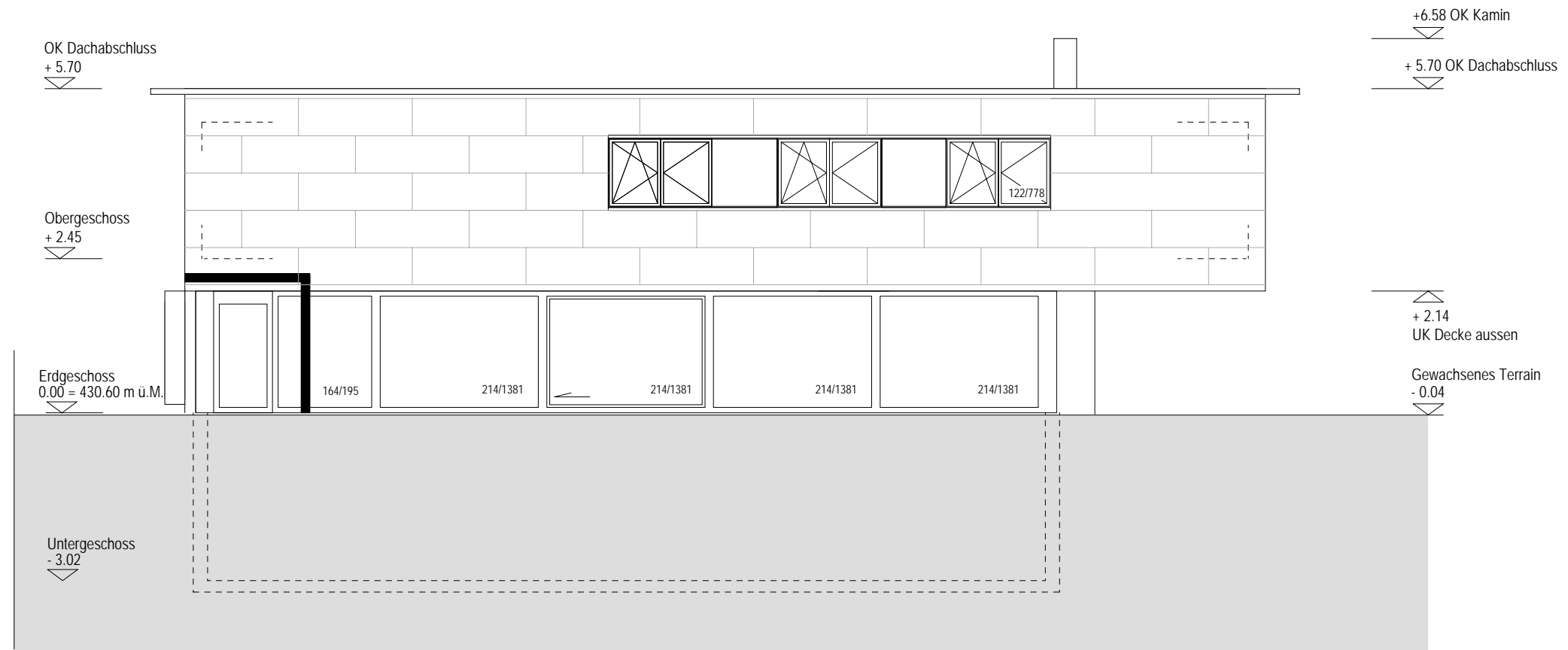
WESTANSICHT
