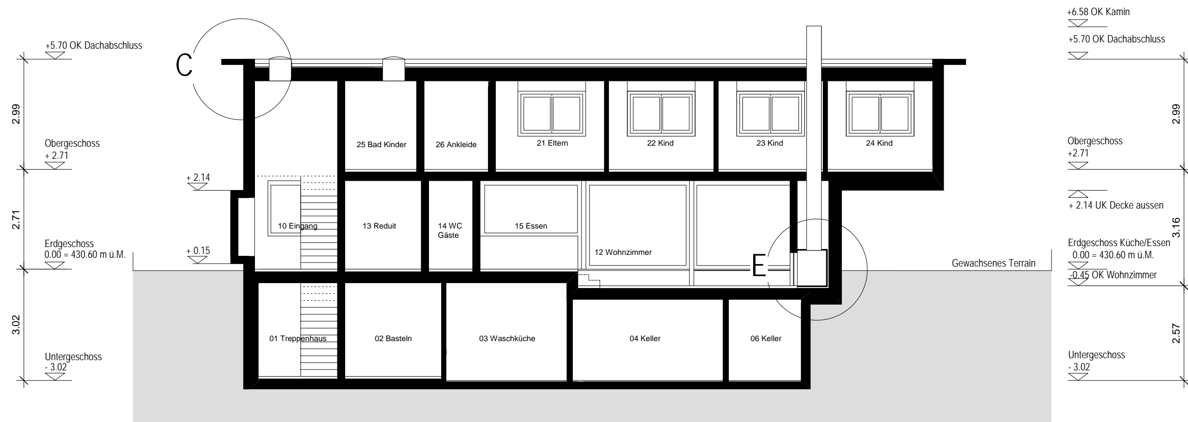
LÄNGSSCHNITT A-A
