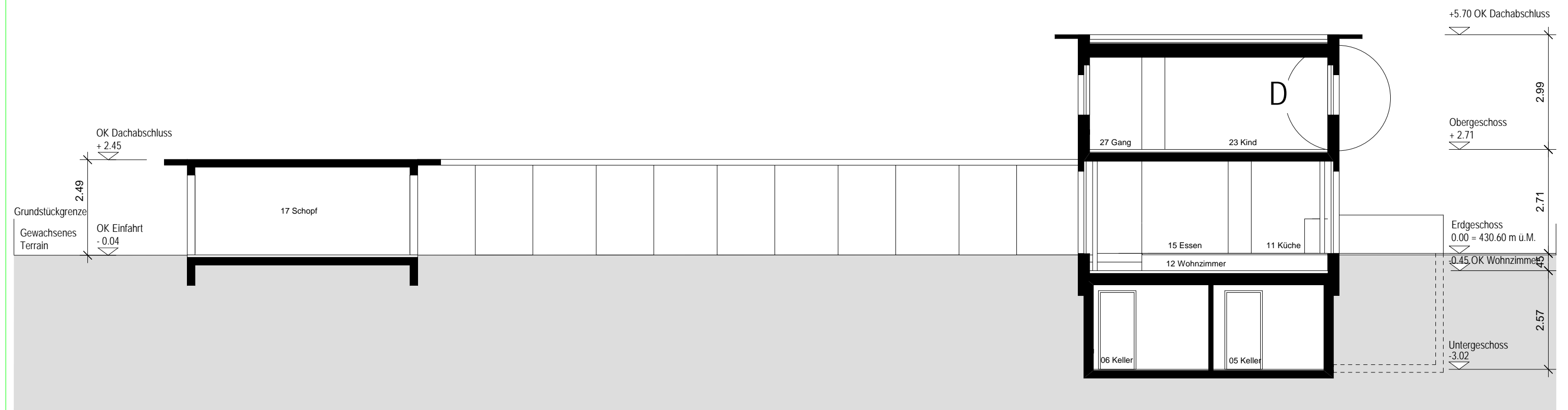
QUERSCHNITT B-B
